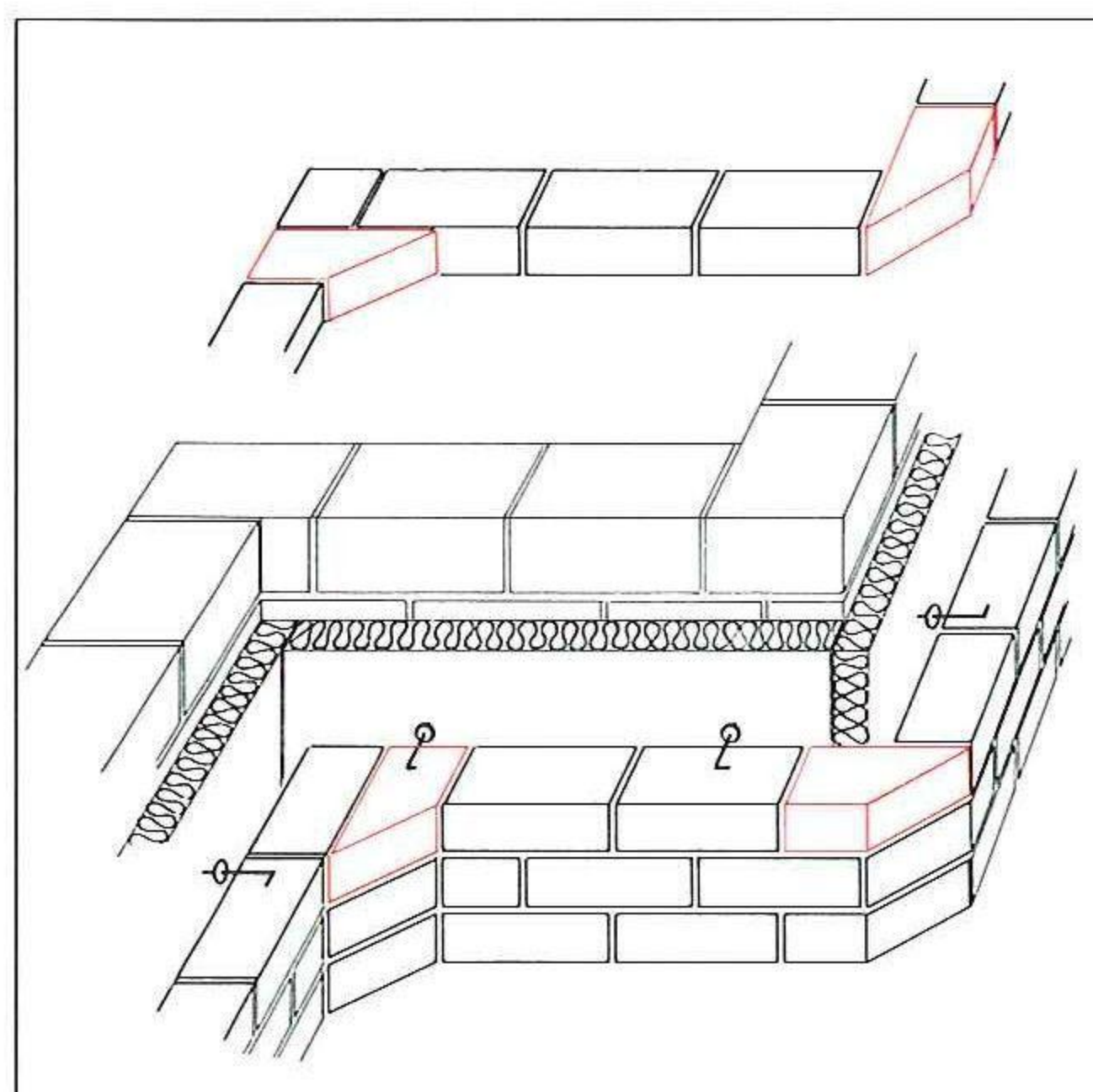
ANWENDUNGSBEISPIEL MAUERECKE
