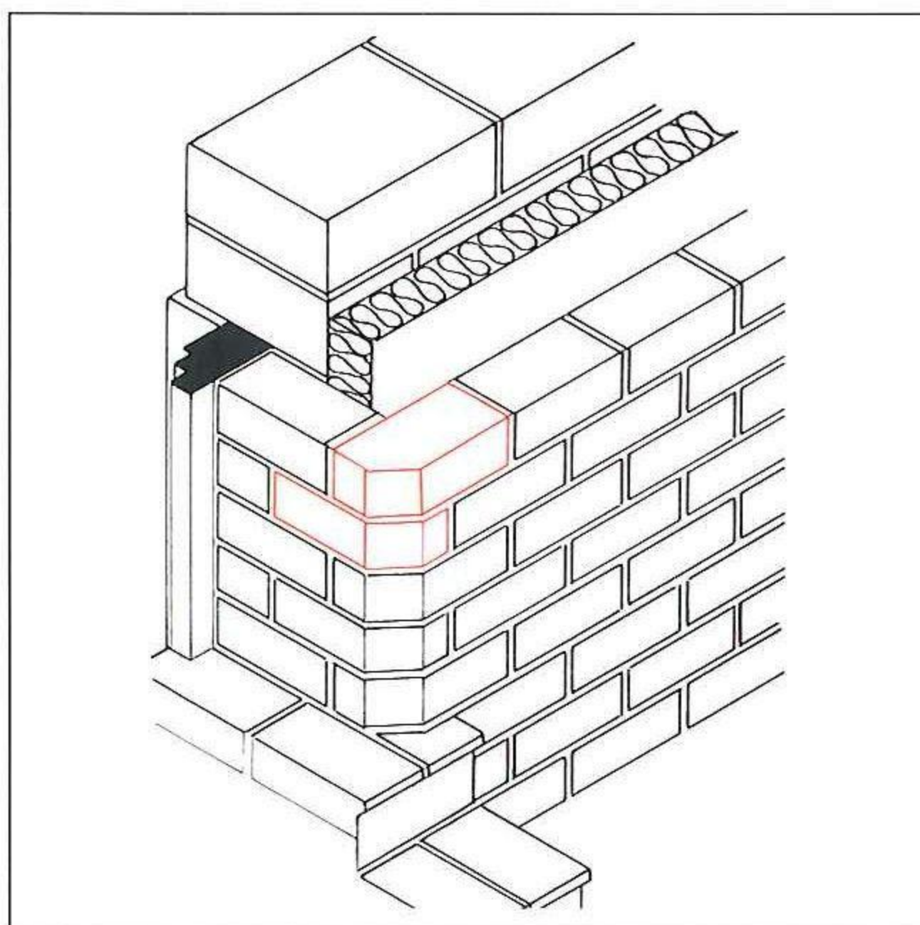
ANWENDUNGSBEISPIEL TÜRLAIBUNG
