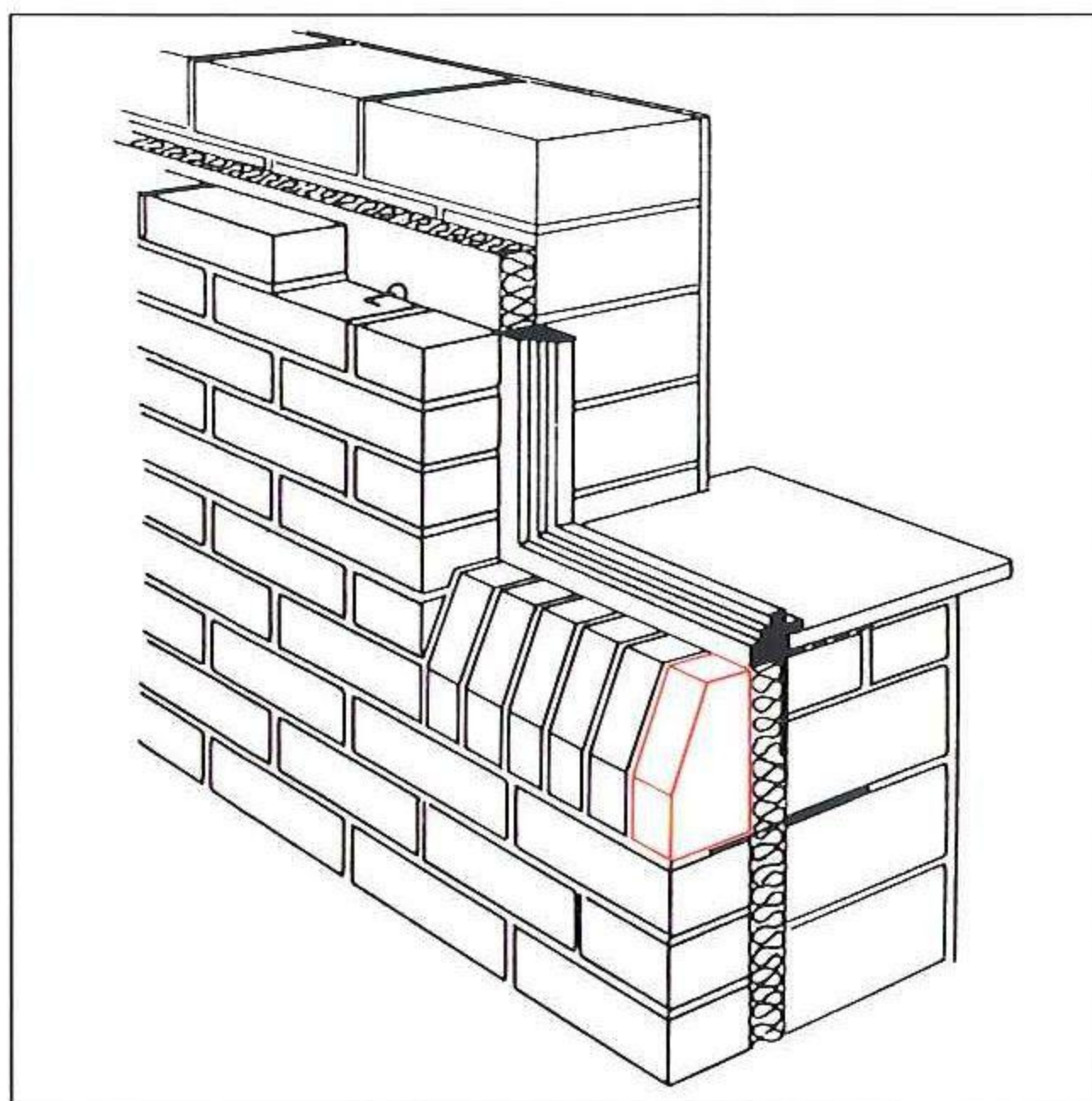
ANWENDUNGSBEISPIEL FENSTERBANK-ABDECKUNG
