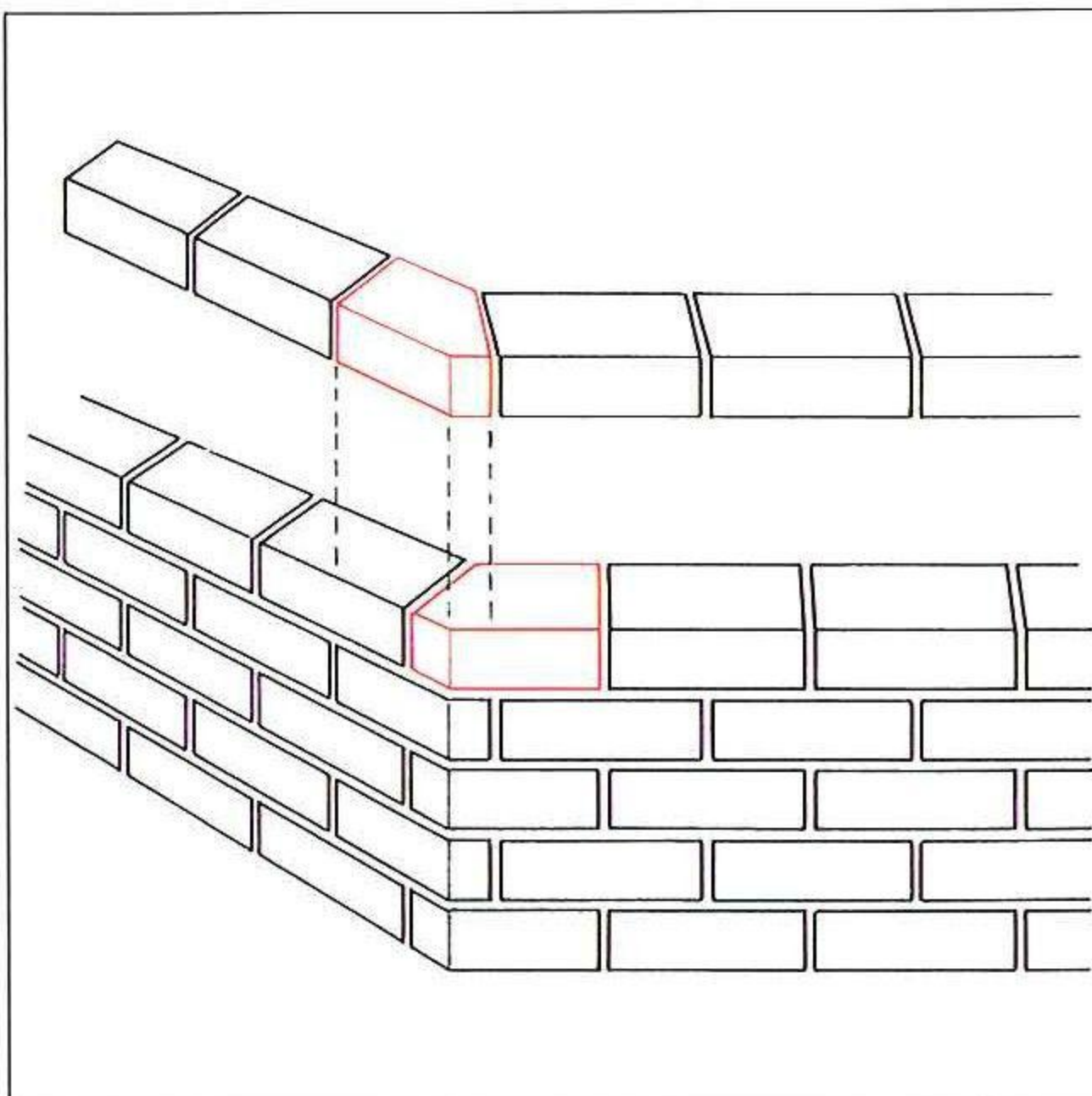
ANWENDUNGSBEISPIEL ECKENAUSBILDUNG
