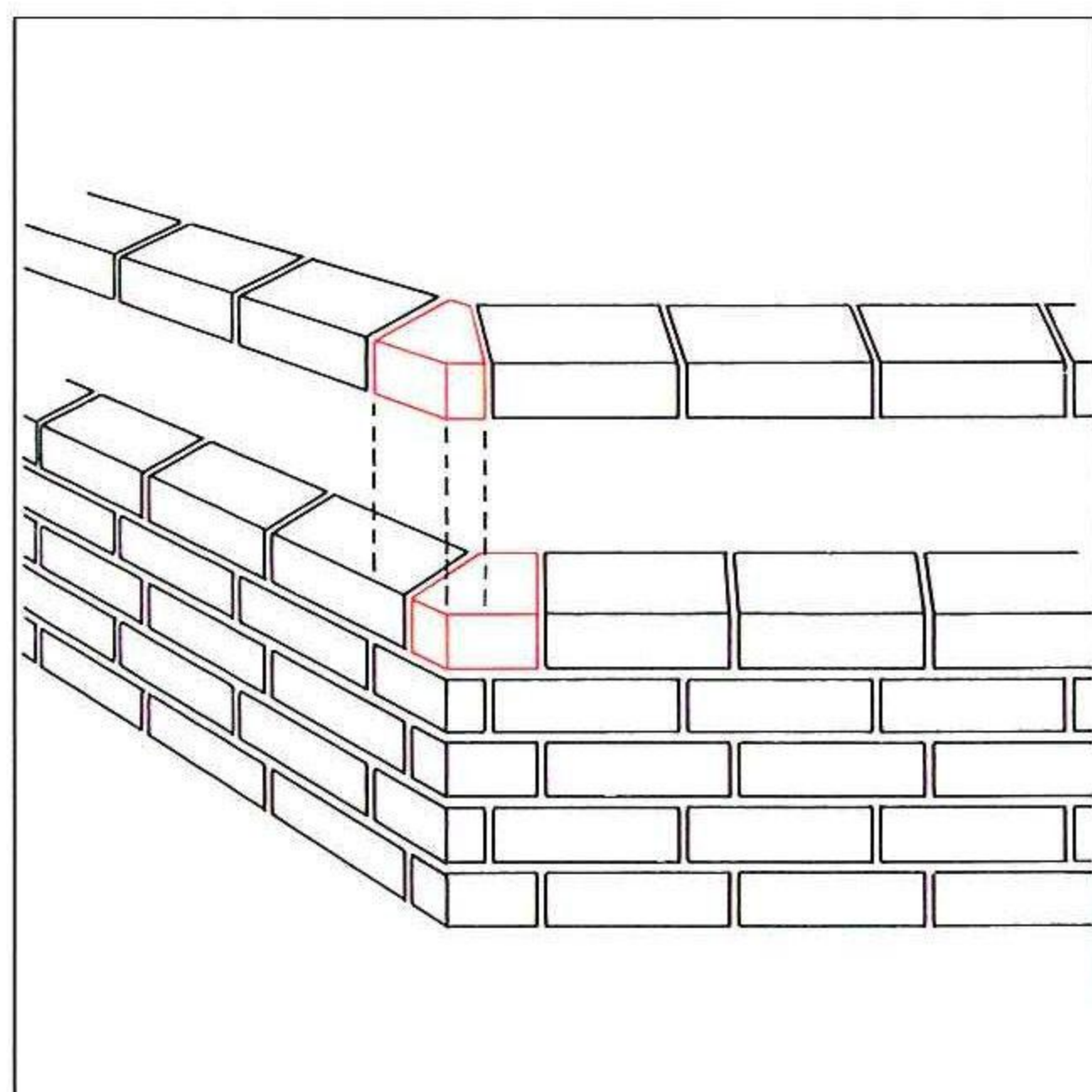
ANWENDUNGSBEISPIEL ECKENAUSBILDUNG 45°
