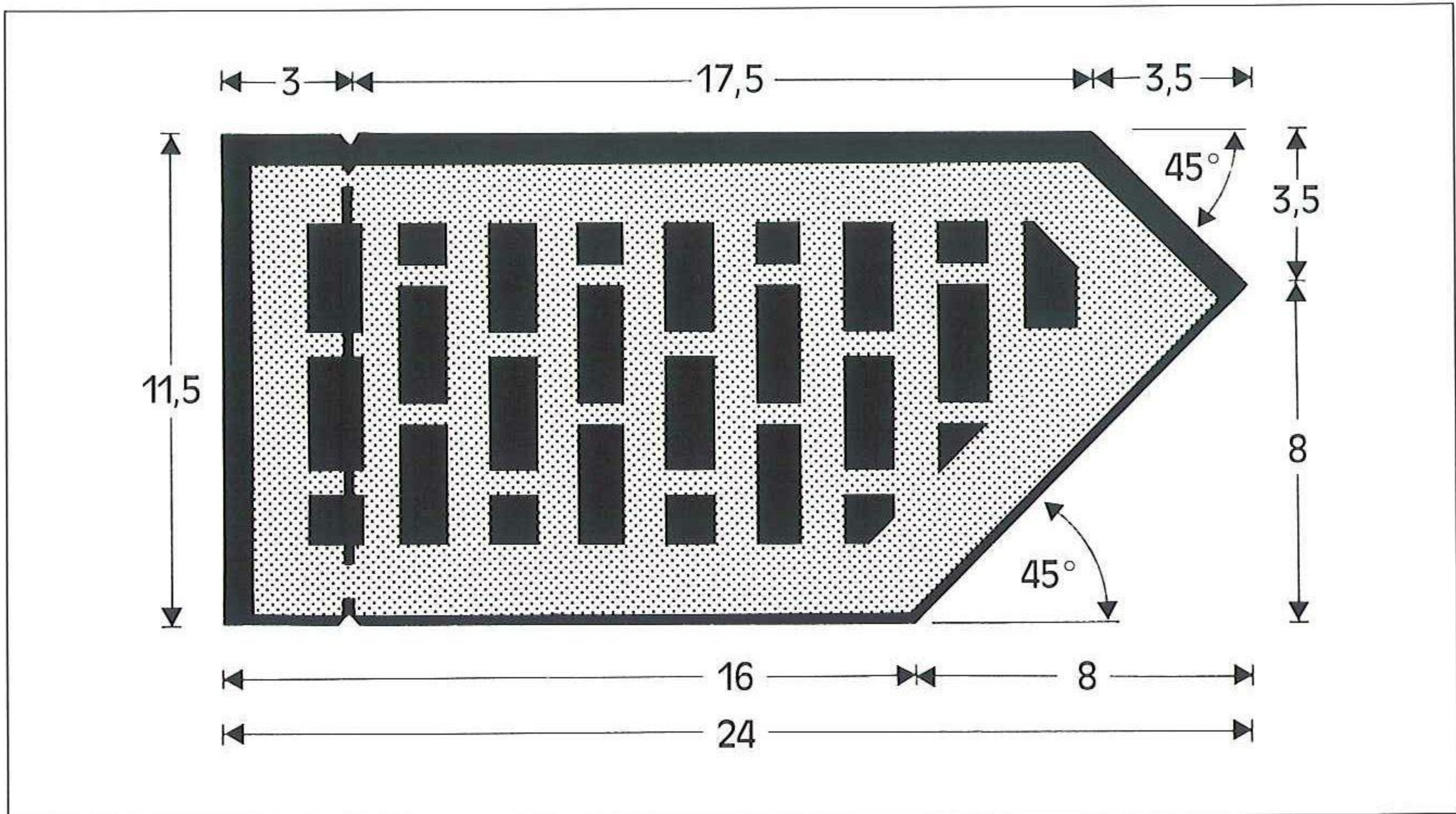
ANWENDUNGSBEISPIEL ECKENAUSBILDUNG
