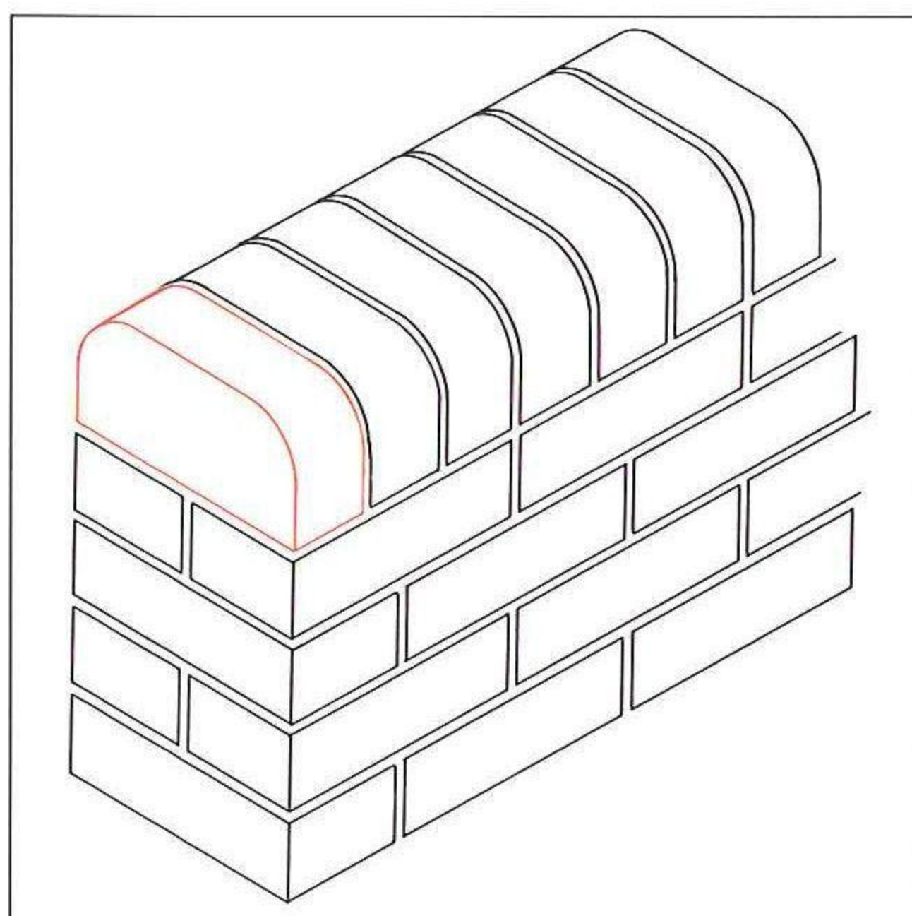
ANWENDUNGSBEISPIEL MAUER-ABDECKUNG
