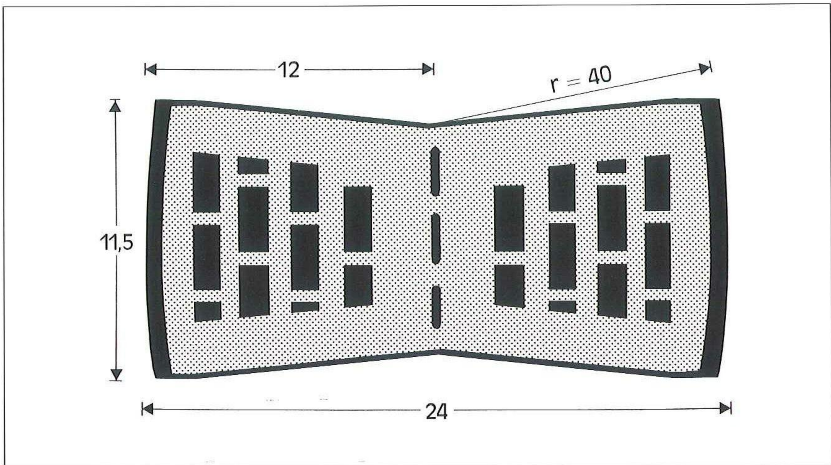
ANWENDUNGSBEISPIEL ECKENAUSBILDUNG
