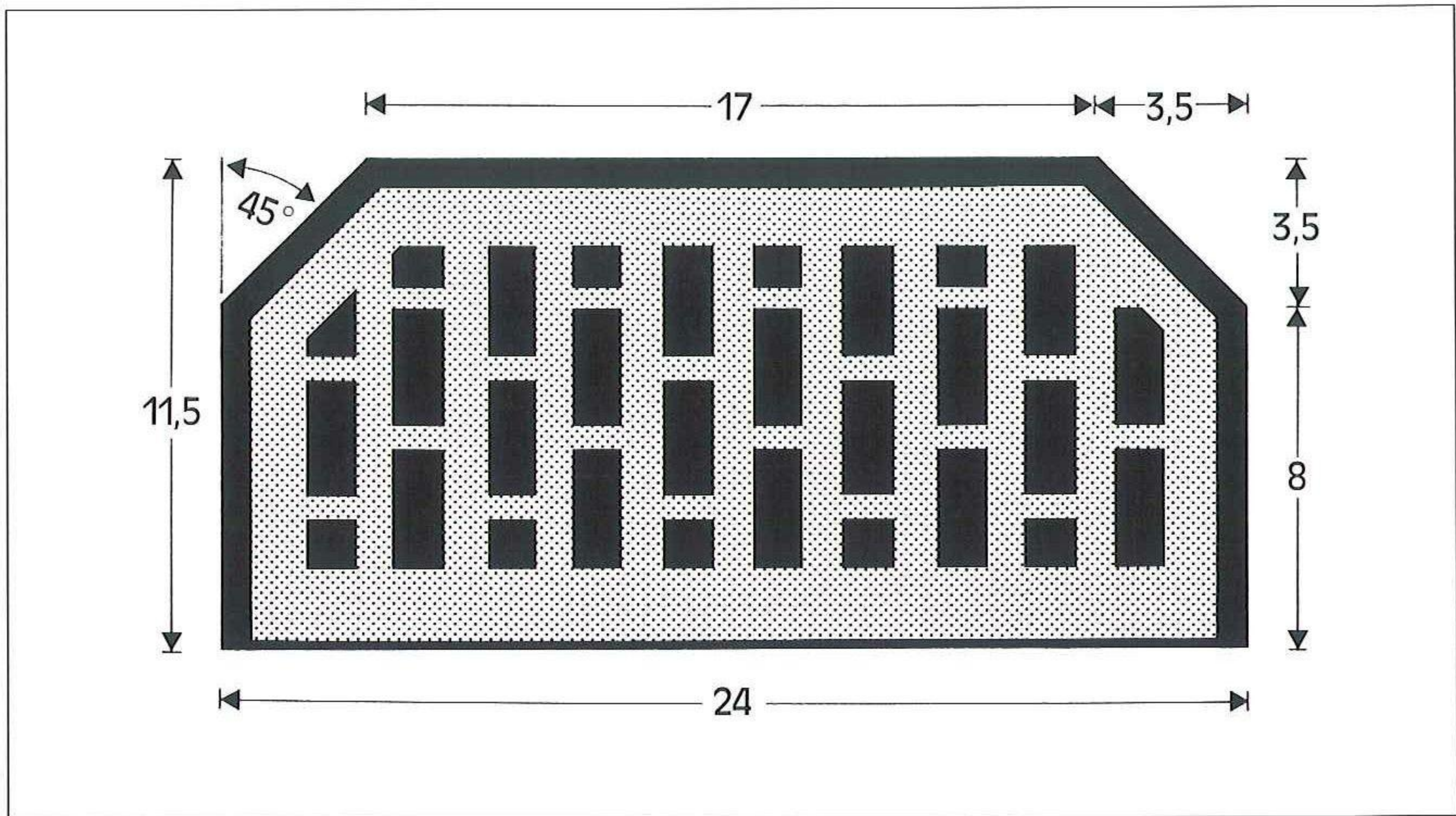
ANWENDUNGSBEISPIEL MAUERABDECKUNG
