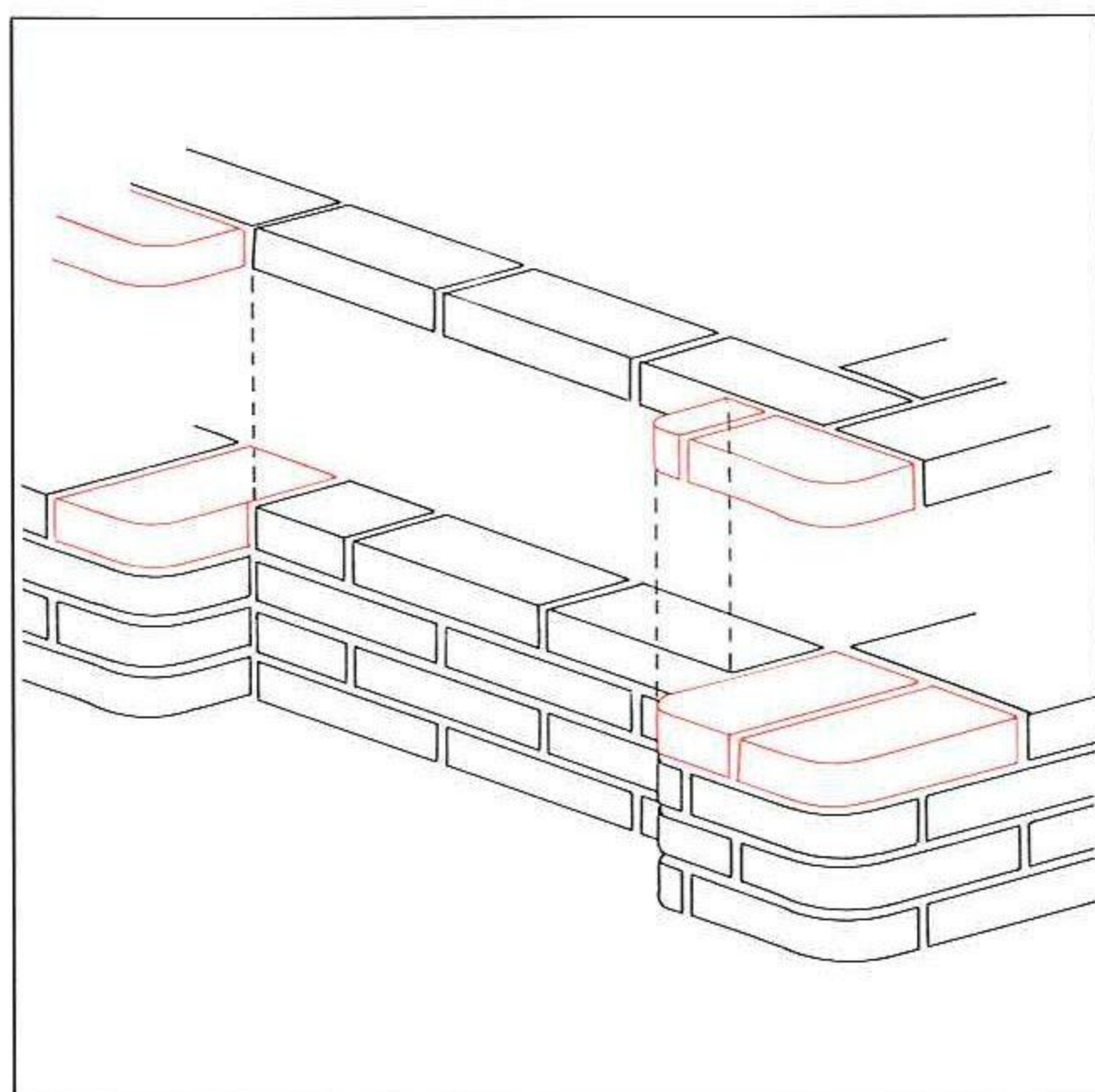
ANWENDUNGSBEISPIEL WANDNISCHEN
