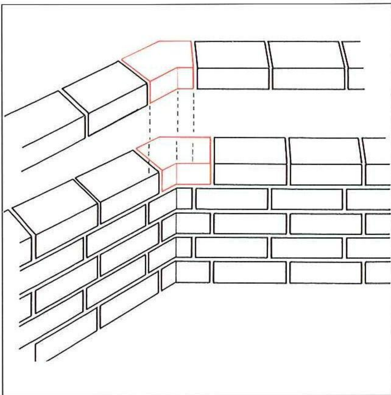
ANWENDUNGSBEISPIEL INNENECKEN 135°
