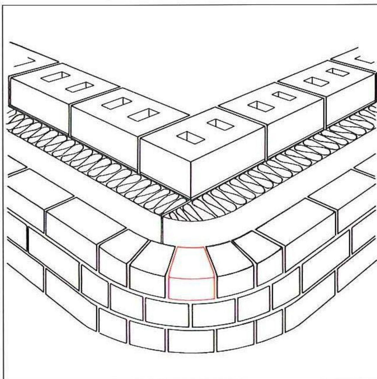
ANWENDUNGSBEISPIEL ECKENAUSBILDUNG
