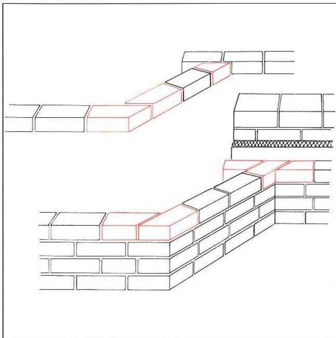
ANWENDUNGSBEISPIEL BALKONBRÜSTUNG
