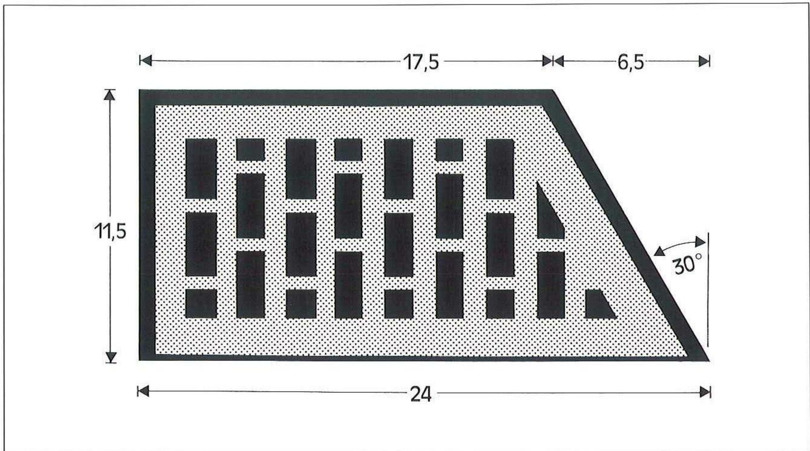
ANWENDUNGSBEISPIEL BALKONBRÜSTUNG
