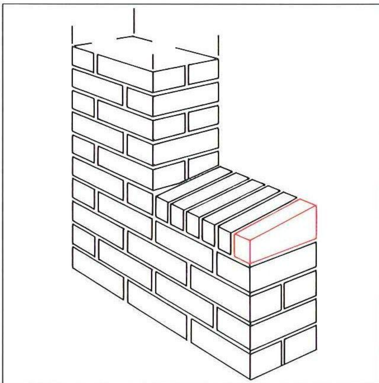
ANWENDUNGSBEISPIEL MAUERABDECKUNG
