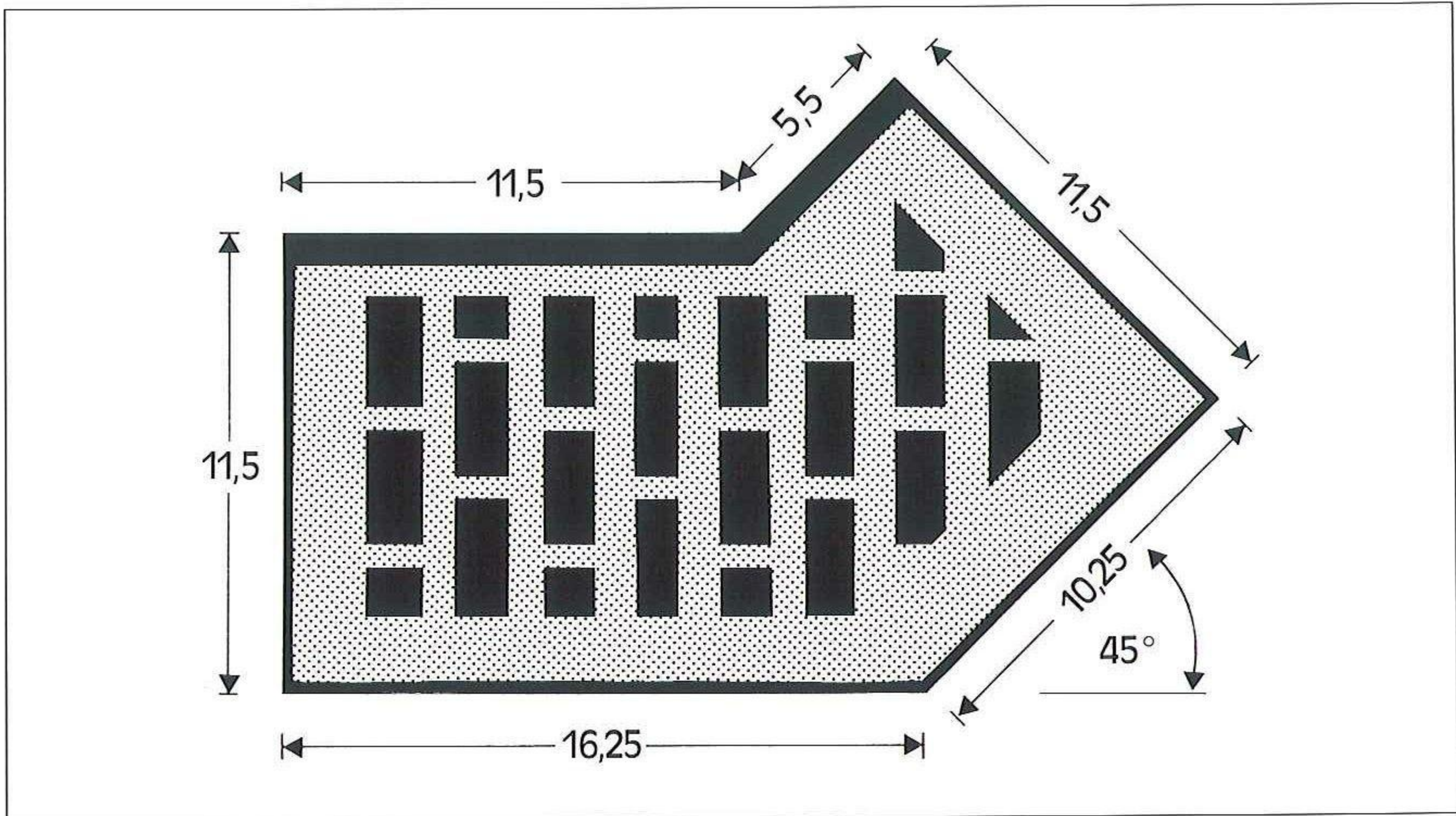
ANWENDUNGSBEISPIEL INNENECKEN 135°
