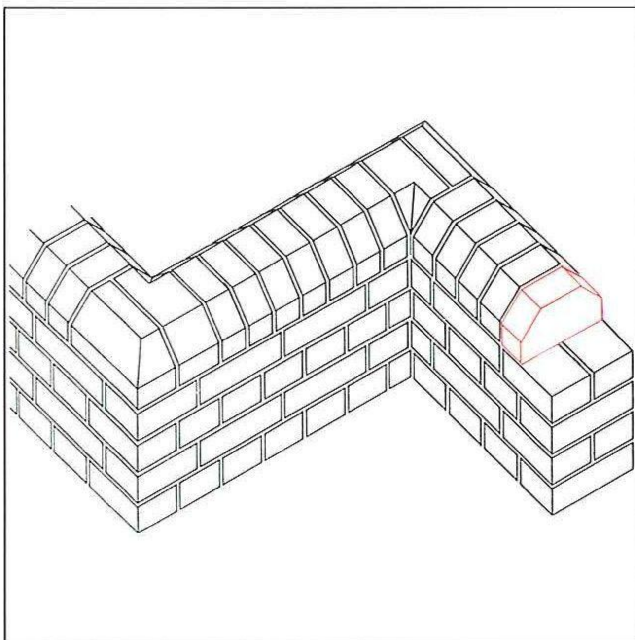
ANWENDUNGSBEISPIEL MAUERABDECKUNG
